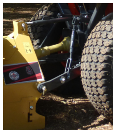
Universele 3de punts aansluiting Attelage universelle
