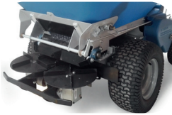
TOPDRESSER Mechanisme met 2 draaischijven
